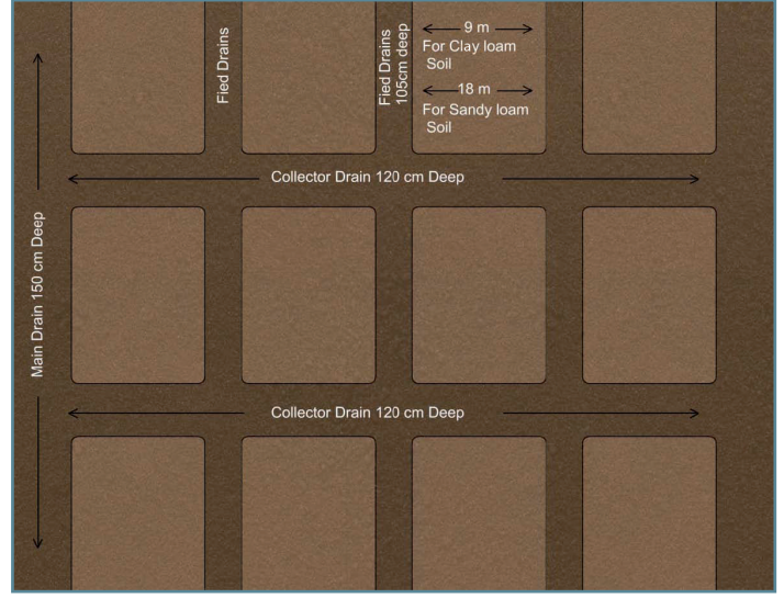
வடிகால் அமைப்பின் திட்டப்படம்
