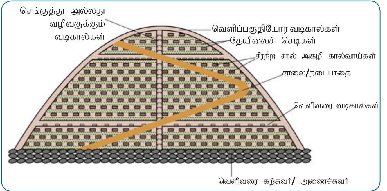
வடிகால் அமைப்பு
