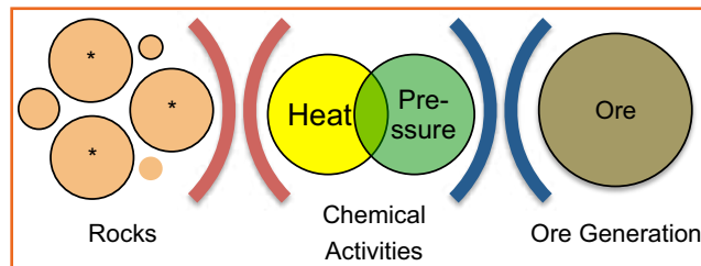
Fig. 1.1.8 Formation of ores
